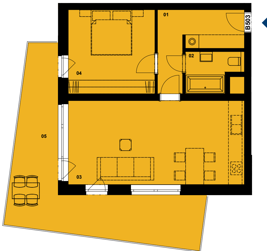
PŮDORYS 5.NP UMÍSTĚNÍ BYTOVÉ JEDNOTKY V RÁMCI PODLAŽÍ
