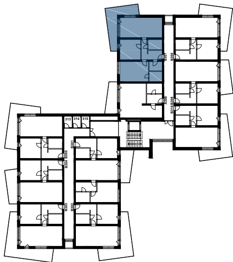
PŮDORYS 3.NP UMÍSTĚNÍ BYTOVÉ JEDNOTKY V RÁMCI PODLAŽÍ
