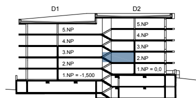
ŘEZ
